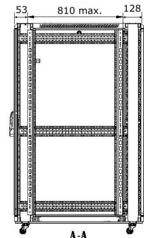
A-A
